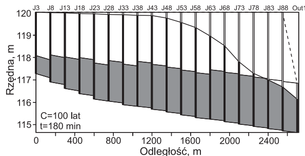
Rys. 10. Profil kolektora w 60. minucie trwania deszczu modelowego Fig. 10. Interceptor profile in the 60 th minute of the model rainfall
